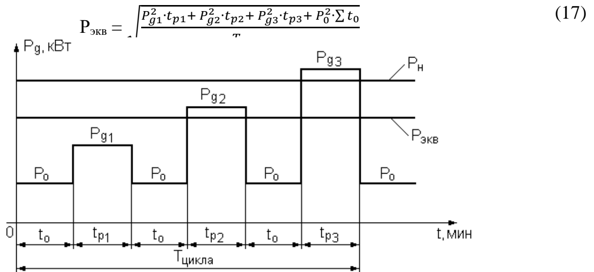
Рисунок 2 Нагрузочная диаграмма
